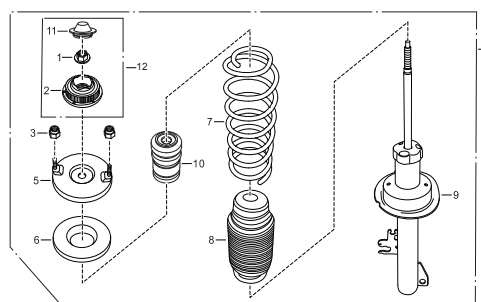
左前弹簧减振器总成
