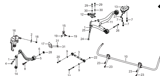
左后悬架
