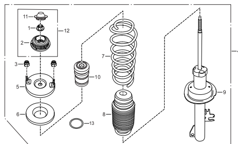
右前弹簧减振器总成
