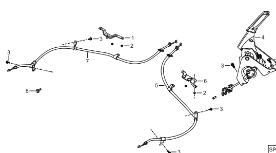
驻车制动系统
