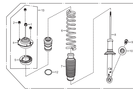
左后弹簧减振器总成
