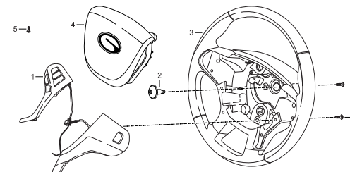
方向盘
