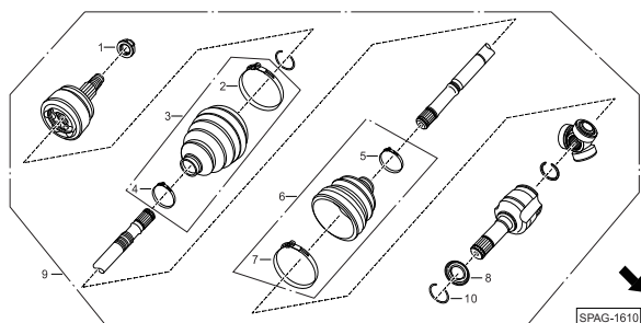
左前驱动轴总成
