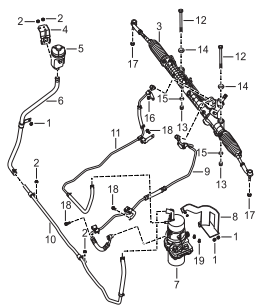
电液动力转向系统
