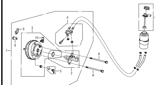
真空助力器附件
