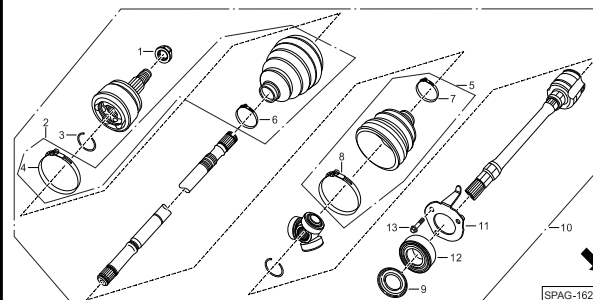
右前驱动轴总成
