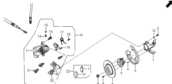
左后制动器总成
