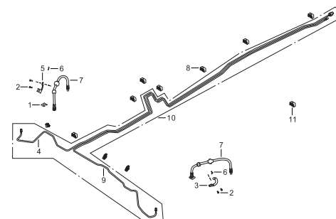
制动管路系统-1
