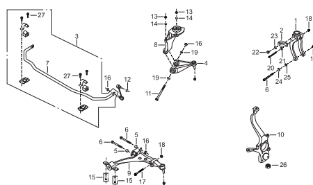
右前悬架
