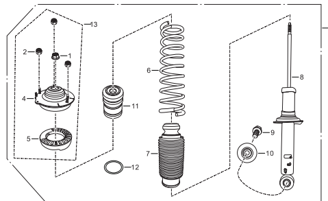
右后弹簧减振器总成
