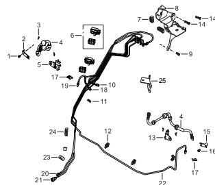
制动管路系统-2
